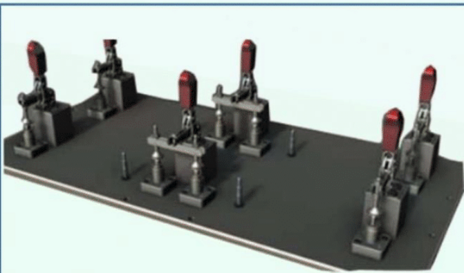
Đồ gá hàn Welding Jig
