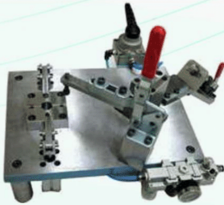
Đồ gá kiểm tra chi tiết Inspection Jig for part
