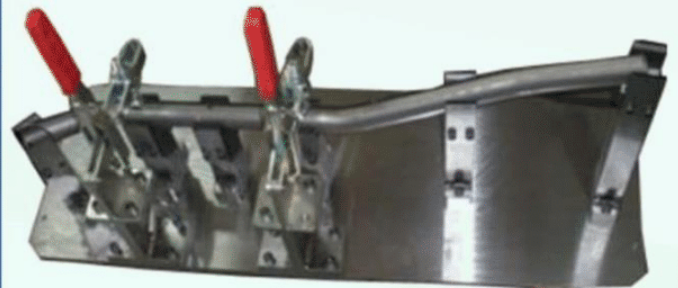
Đồ gá kẹp chi tiết cho gia công Clamping Jig for machining
