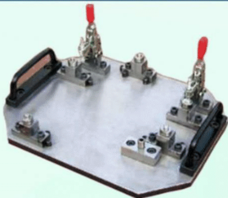
Đồ gá kiểm tra chi tiết Inspection Jig for part
