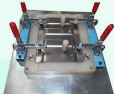
Đồ gá kiểm tra chi tiết Inspection Jig for part
