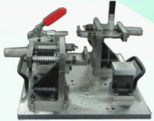
Đồ gá kiểm tra chi tiết Inspection Jig for part
